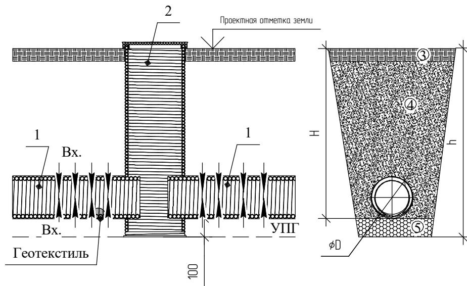
Рис.4 Дренажная горизонтальная система отведения вод Вх. - вход воды в дренажные трубы; 1. Труба дренажная ТД марки "ВИТАЛ", 2. Колодец смотровой КДС 3. Слой почвы, 4. Засыпка песком, 5. Подушка-гравий/щебень.
