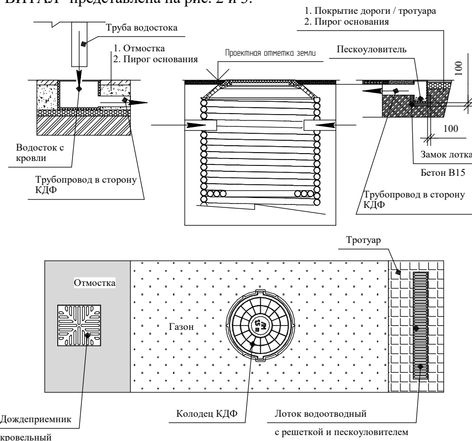
Рис.2 Локальная автономная система отведения поверхностных ливневых и талых вод
